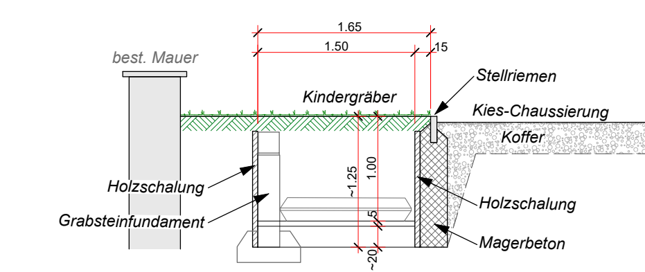
Schnittansicht B-B 1:50 Kindergräber
